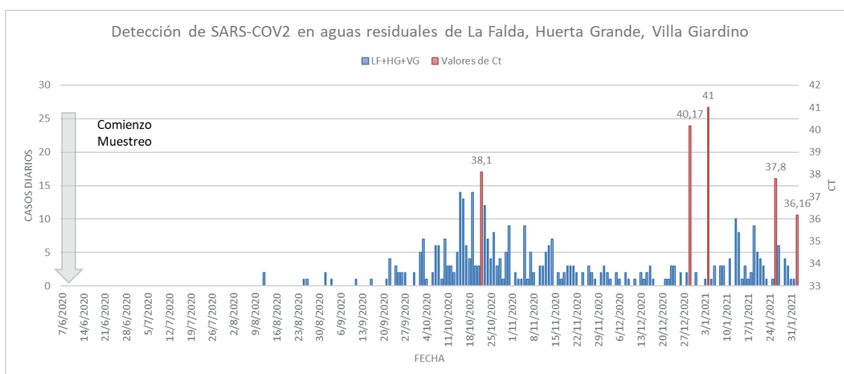
Figura 3. Primera detección de SARS-CoC-2 en la planta de tratamiento de aguas residuales que reúne a la localidad de La Falda, Villa Giardino y Huerta Grande.
