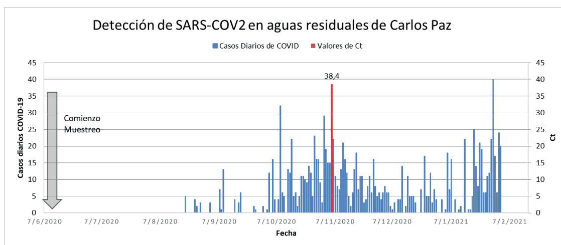
Figura 4. Primera detección de SARS-CoC-2 en aguas residuales de Costa Azul, Carlos Paz.
