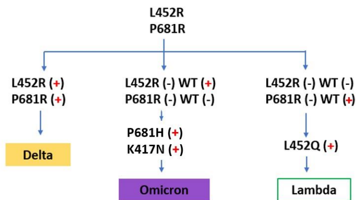
Figura 1. Estrategia de detección de variantes mediante RT-PCR en tiempo real utilizando el reactivo TaqMan™ SARS-CoV-2 Mutation Panel (Applied Biosystems), para la detección de mutaciones relevantes en VOC y VOI, implementada en el Laboratorio Central, acorde a las variantes de circulación actual.
